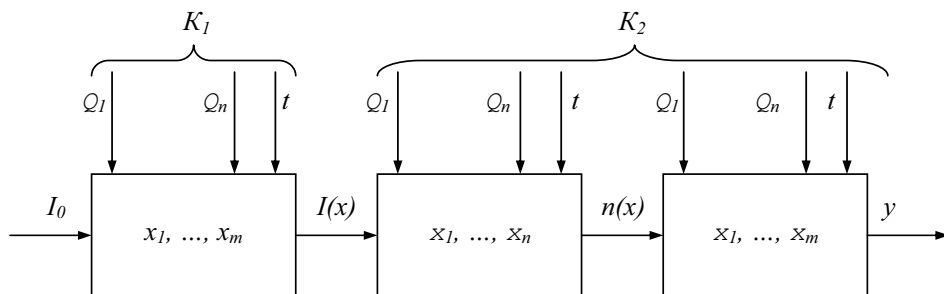
Рисунок. Обобщённая функциональная схема прямого измерения
